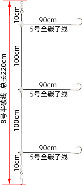
主线和子线连接采用十字交叉豆 360度无阻碍自由回转，杜绝缠绕
